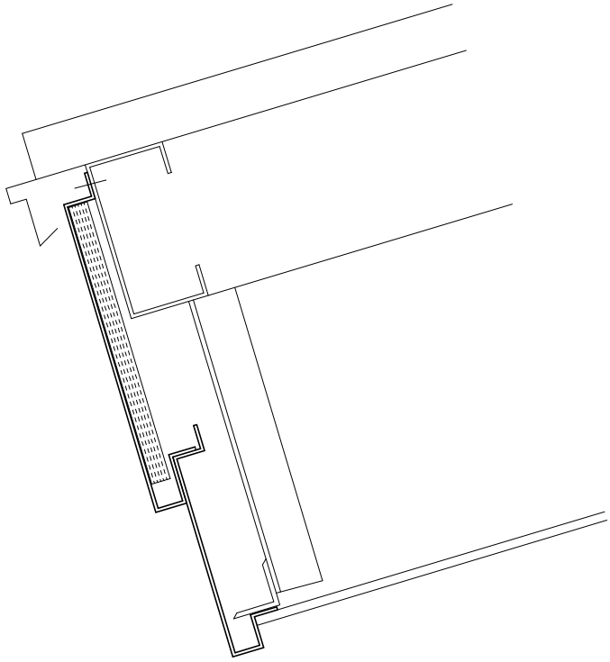
軒先 樋取付け部
